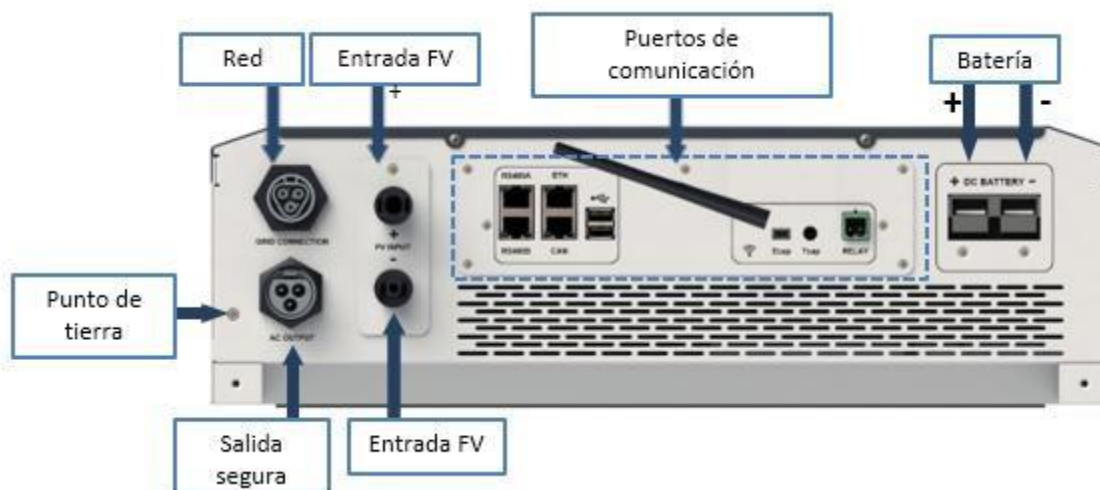
N 3.6: Descripción de las conexiones disponibles
