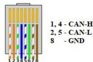
Figura - Cableado RJ45
